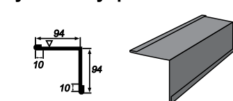
Кутник внутрішній
