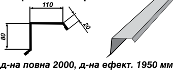
Вітрівниця верхня
