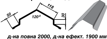
Коньок трапецієвидний
