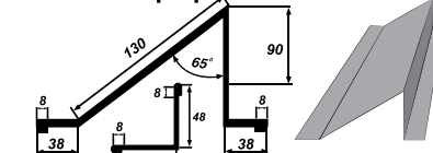
Сніговий бар'єр
