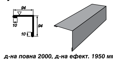
Кутник зовнішній
