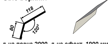
Звіс верхній
