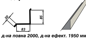
З'єднувач малий
