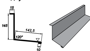
З'єднувач великий
