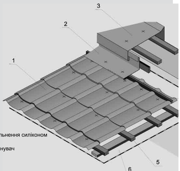
Рис. 16. Вузол примикання покрівлі до стіни по торцю
